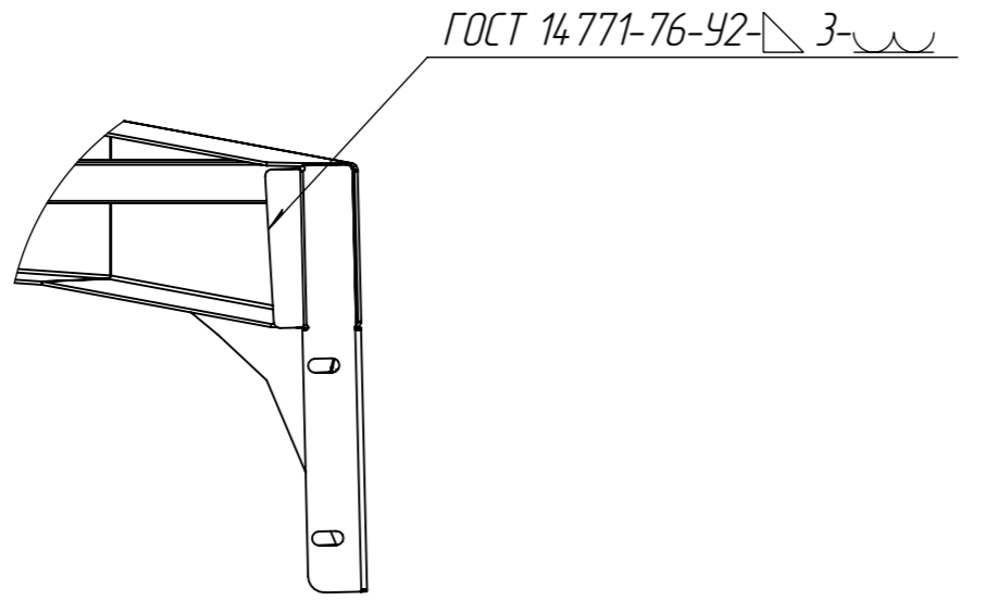
ВИД С МАСШТАБ 1:5
